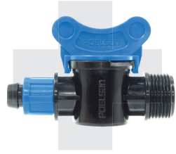
MINI VANA Damlama - Erkek MINI VALVE Dripline - Male
